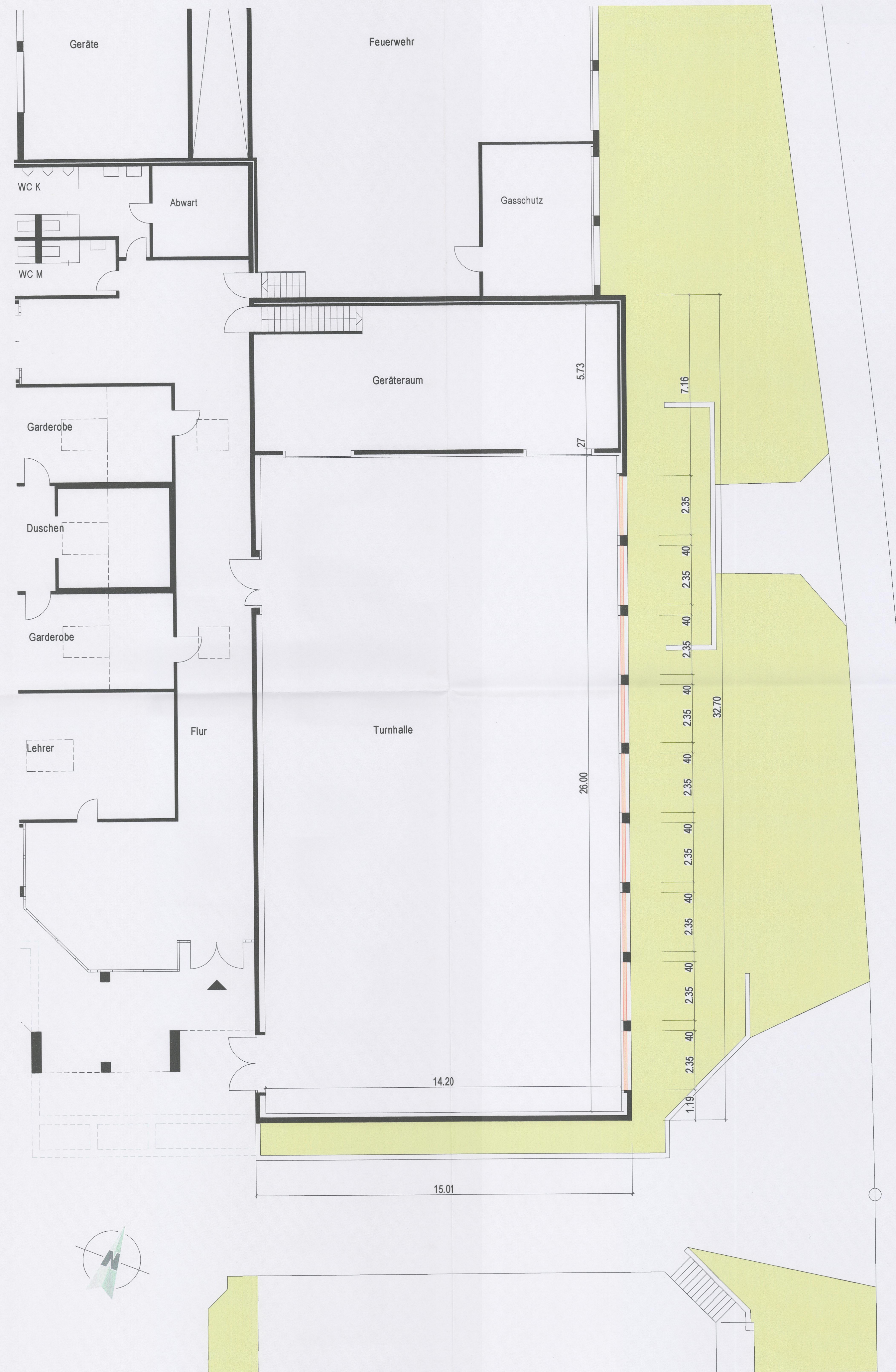
Grundriss
